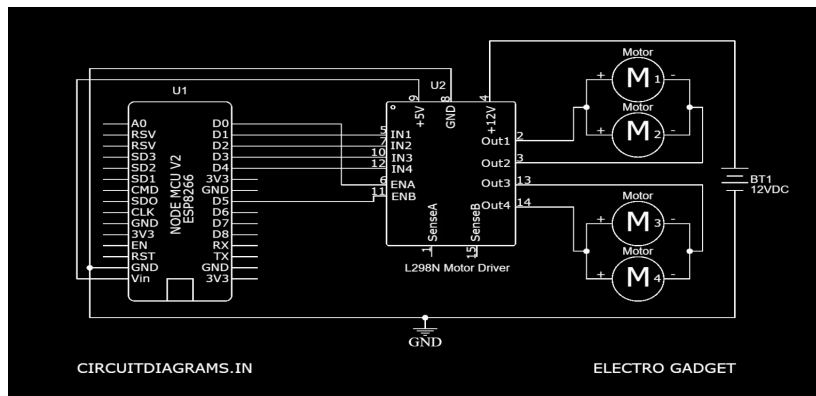
Fig a: Circuit Diagram
